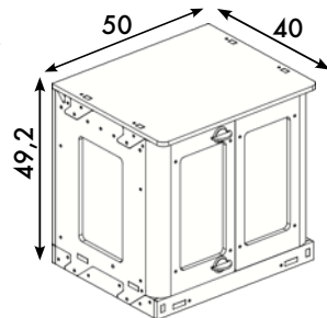
Modulo contenitore 40 Alto
