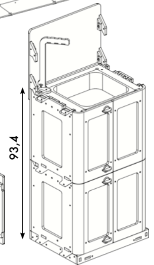
Modulo Lavello 40 Doppio
