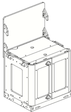
Modulo porta fornello 40 Alto
